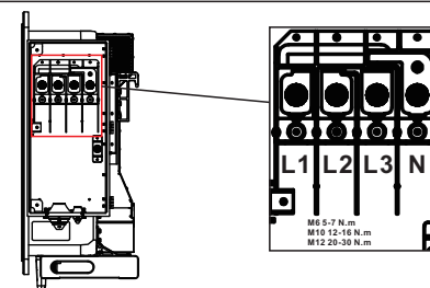
图3.22 交流端子排
